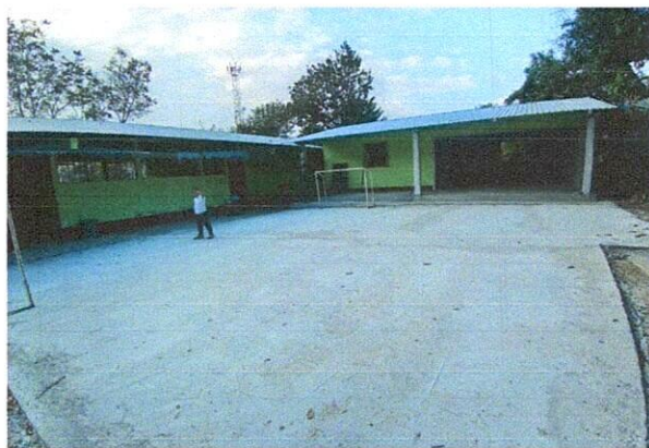
Foto 2: Reparación o sustitución de área de cocina. Sustitución de cubierta de techo y estructura metálica.
